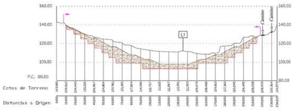
PERFIL T3-T3'
